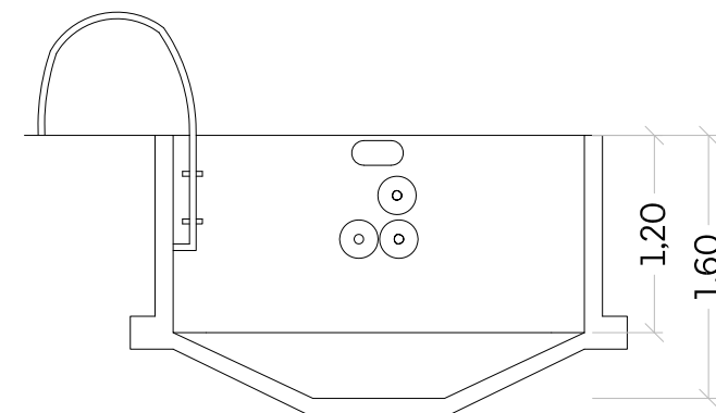
SECCIÓN TRANSVERSAL
