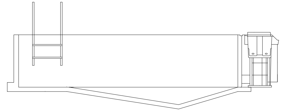
SECCIÓN LONGITUDINAL
