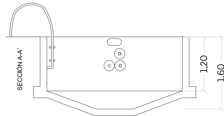
SECCIÓN TRANSVERSAL
