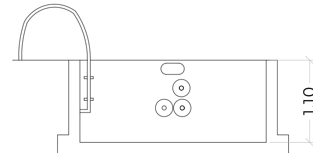
SECCIÓN TRANSVERSAL
