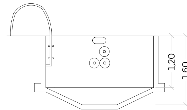
SECCIÓN TRANSVERSAL
